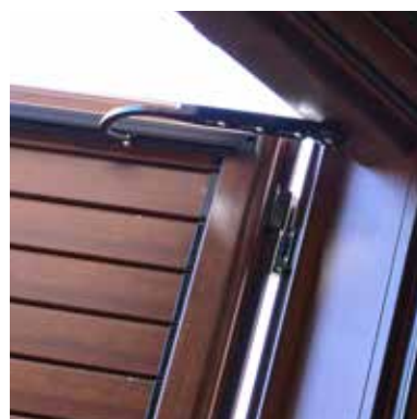
Braccio con apertura elettrica
