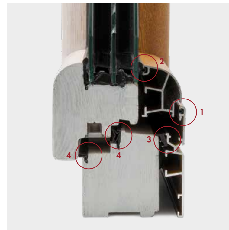
Sezione anta legno/alluminio arrotondato
